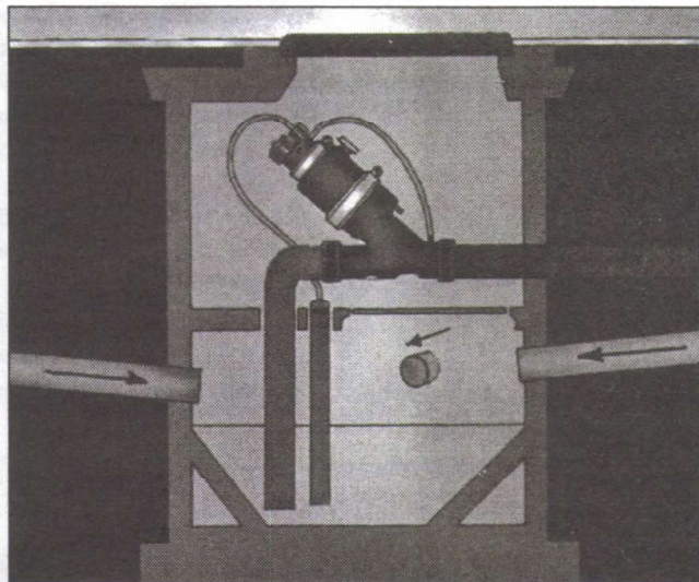
Tipikus gyűjtőakna, 1 m átmérőjű, 2 m mély, vákuumcsatornával és kétoldalt gravitációs házi bekötéssel
