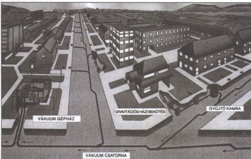
A szennyvíz gyűjtése ISEKI vákuumos rendszerrel
